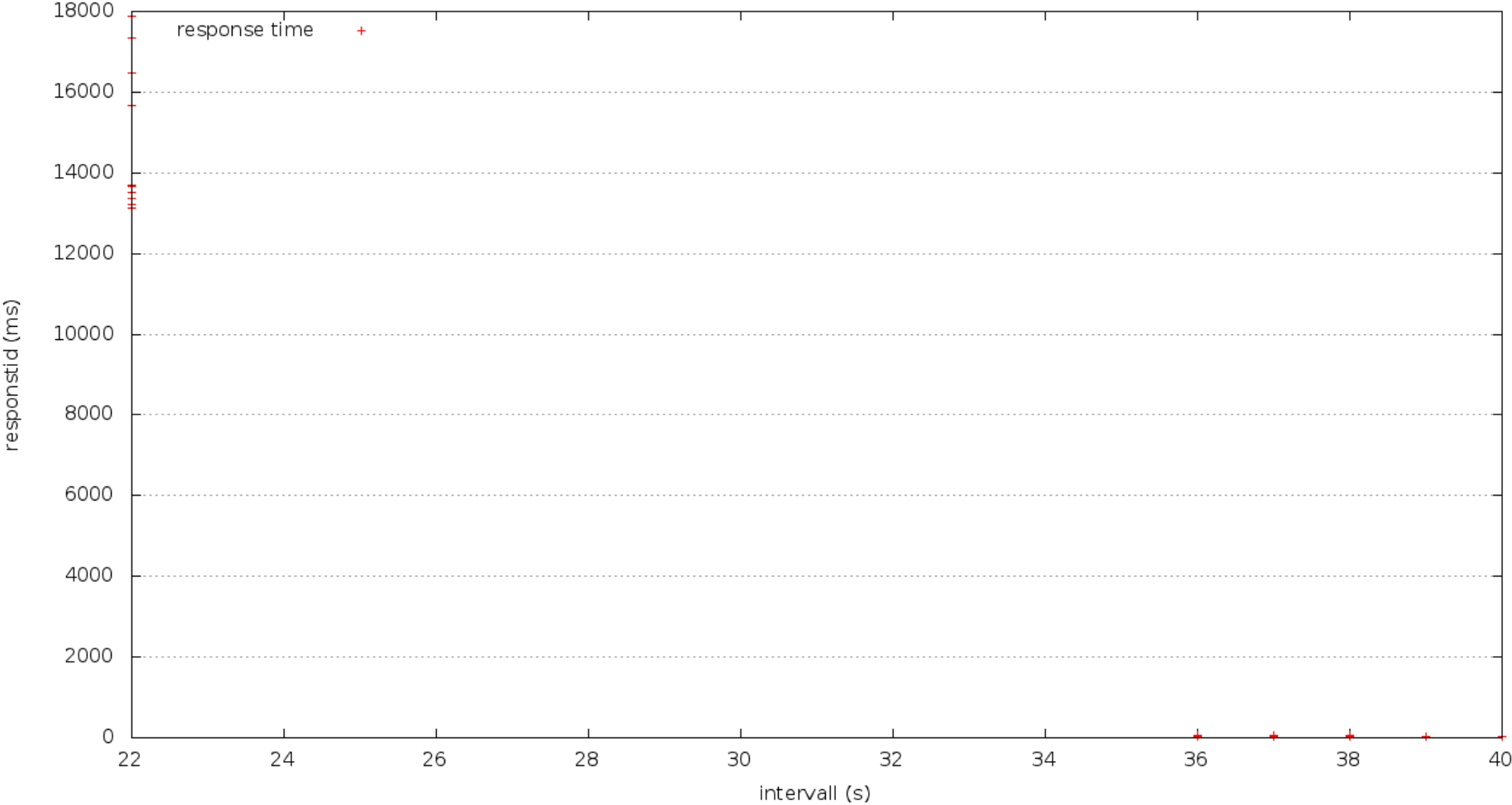
Stresstest: Binerio (med cache)
