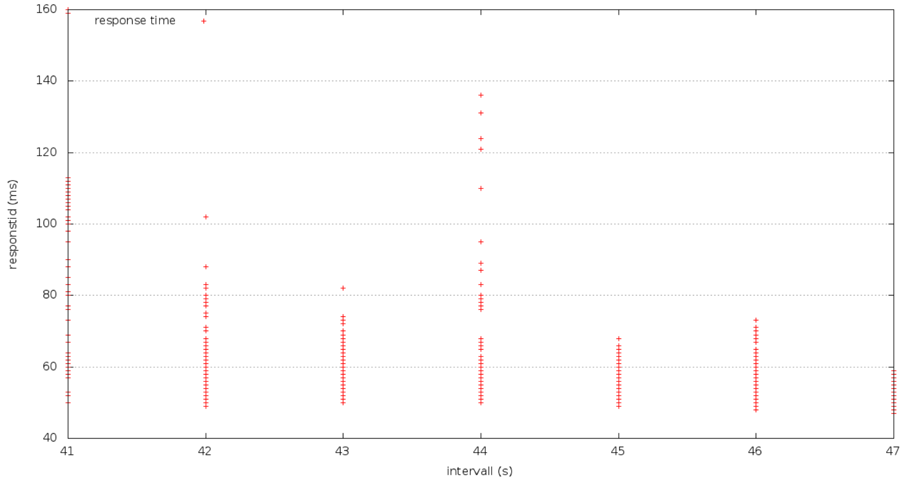
Stresstest: Loopia (med cache)
