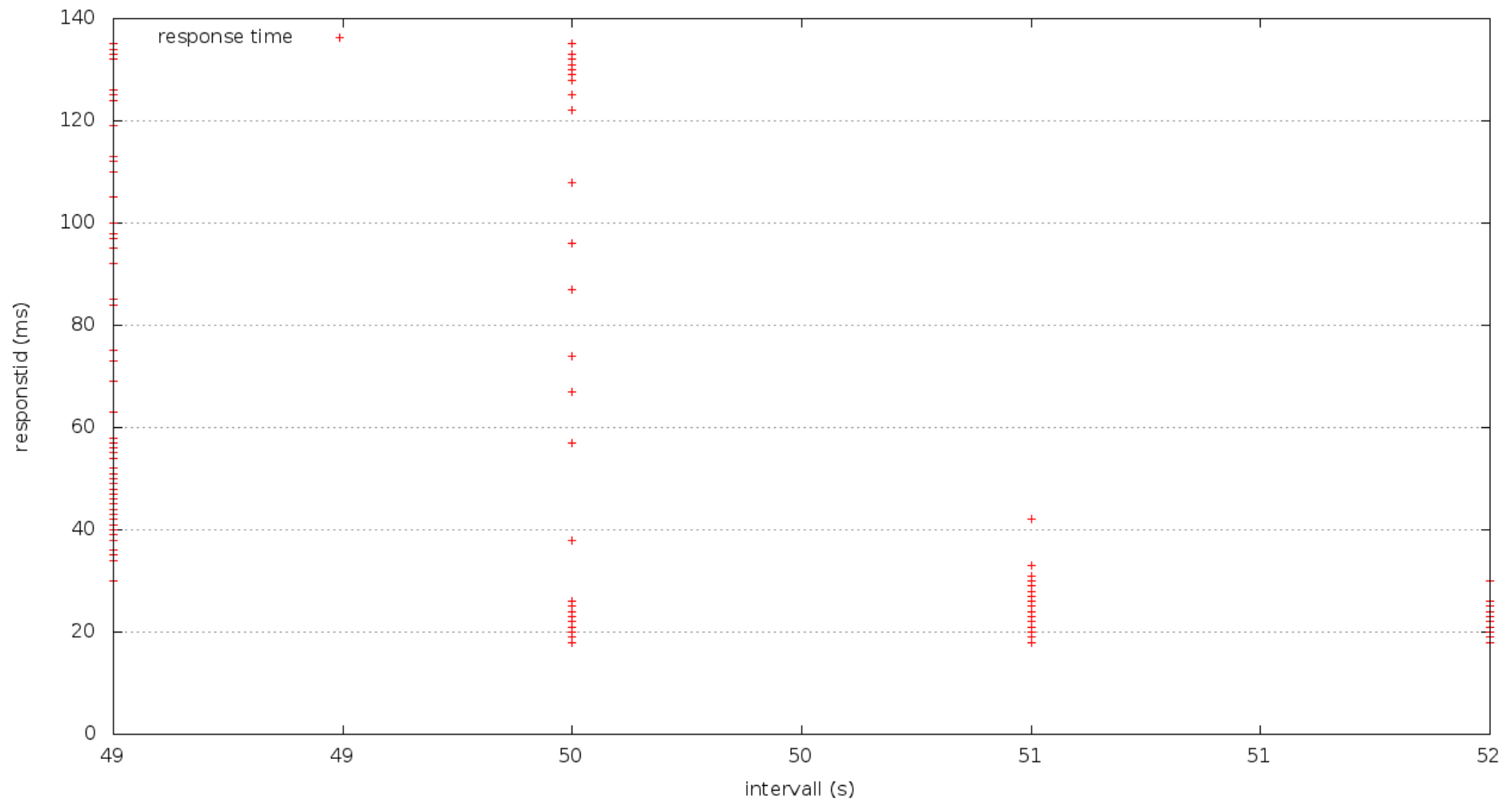
Stresstest: Oderland (med cache)
