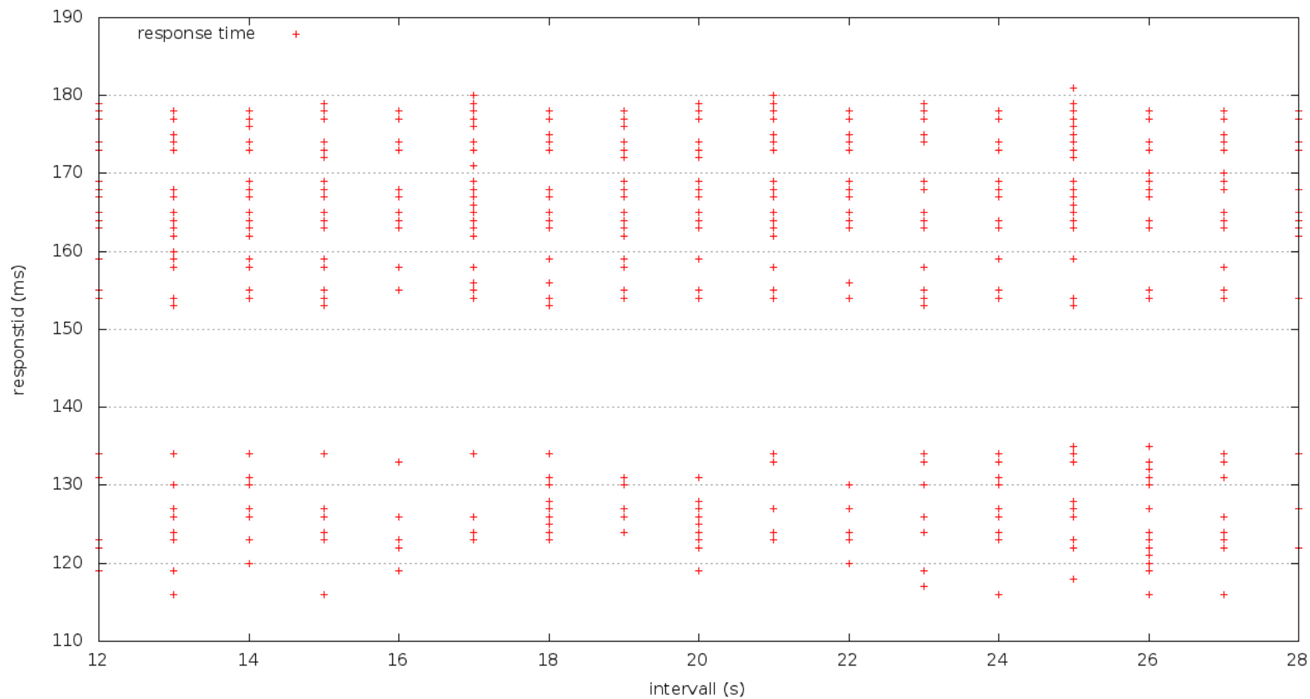
Stresstest: Manufrog (med cache)
