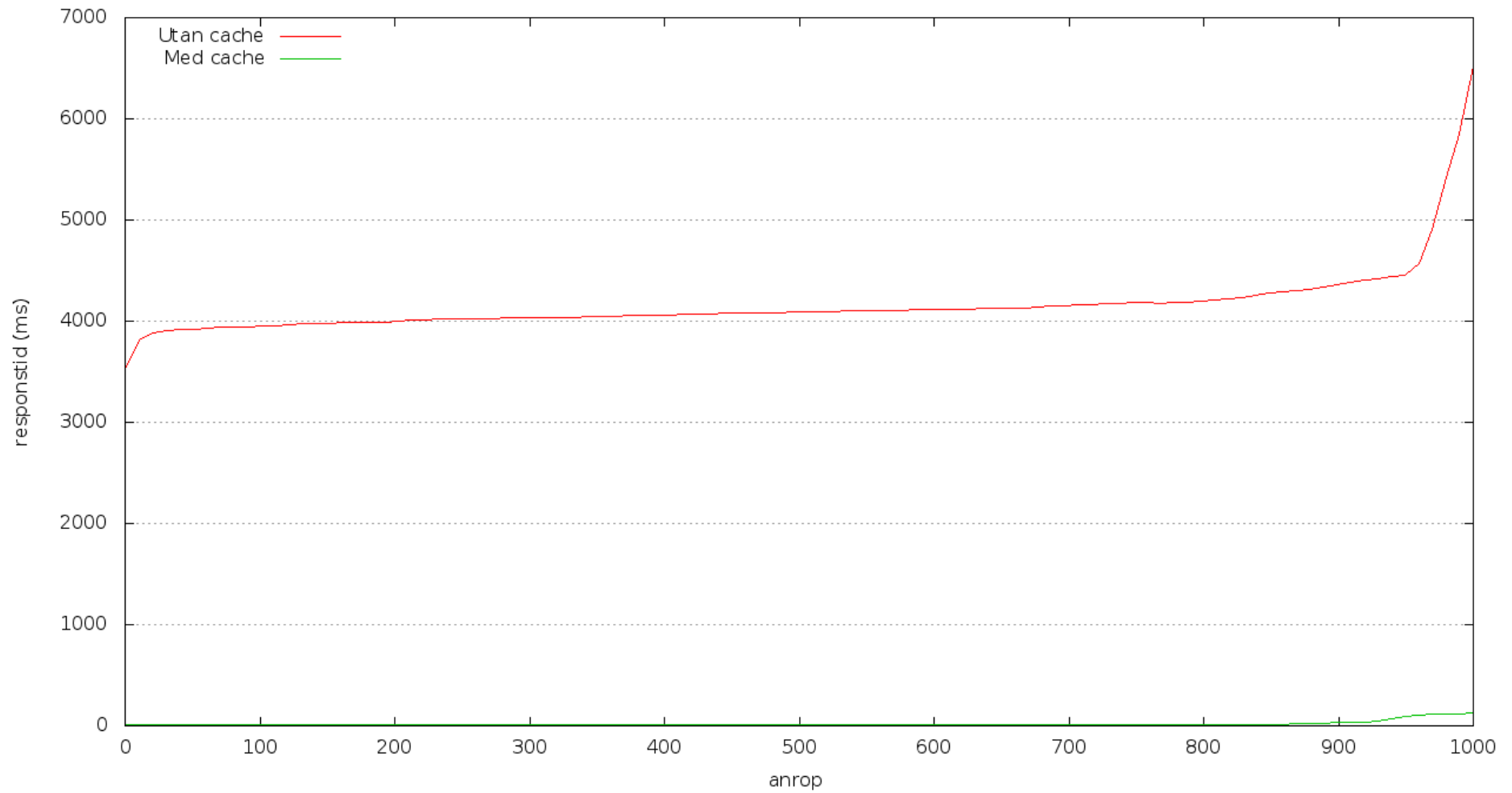
Stresstest: Oderland
